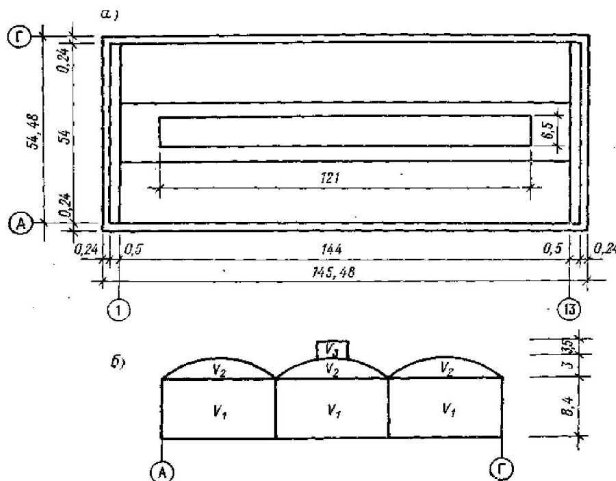
Рис. 29. Определение строительного объема промышленного здания а — план; б — схематический разрез
