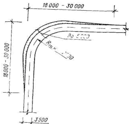
мал . схема розширення дороги при повороті під кутом 90
