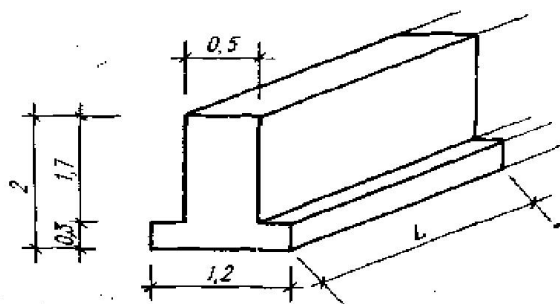
Рис. 28. Определение объема монолитных фундаментов
