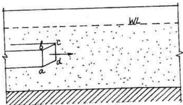
Рисунок 6.8 — Схема визначення дебіту водоносного горизонту
