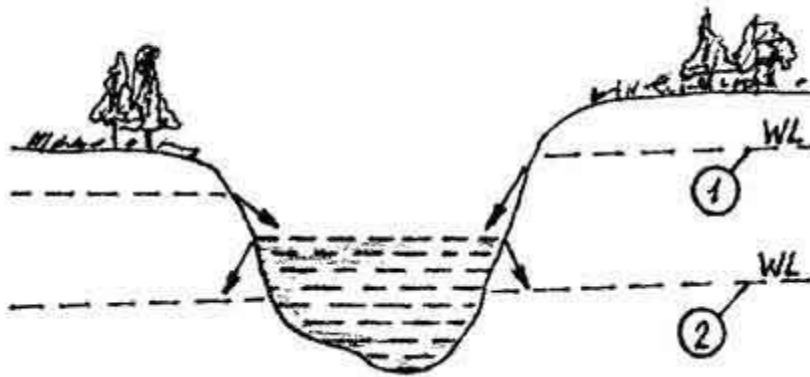
Рисунок 6.7 — Зв'язок між поверхневими та ґрунтовими водами:
