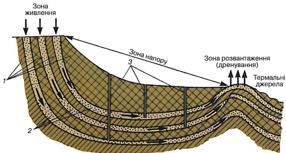
Рисунок 6.6 – Схема будови артезіанського басейну:
