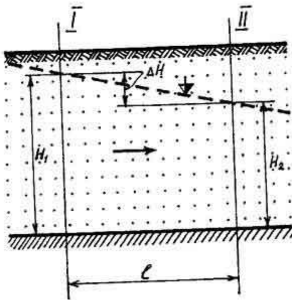
Рисунок 6.9 — Схема руху ґрунтової води
