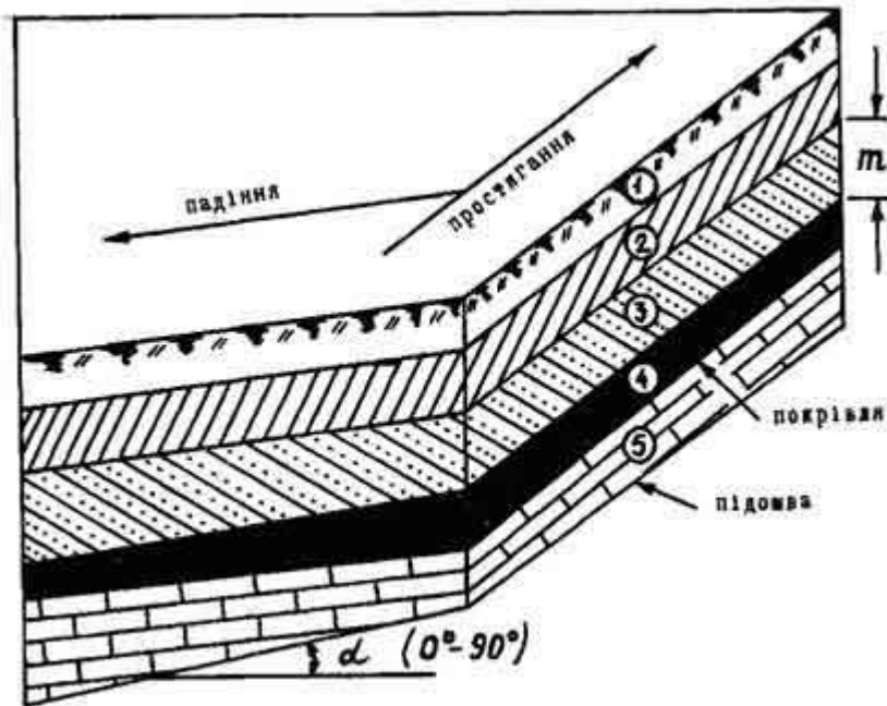
Рис. 5.3 — Форми залягання осадових гірських порід:
