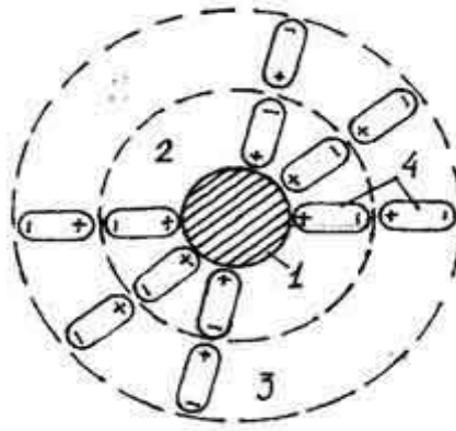
Рисунок 6.2 — Водяні оболонки навколо мінеральної частинки:
