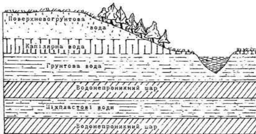
Рисунок 6.4 — Підземні води
