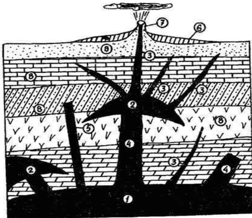
Рисунок 5.1 — Форми залягання магматичних гірських порід:
