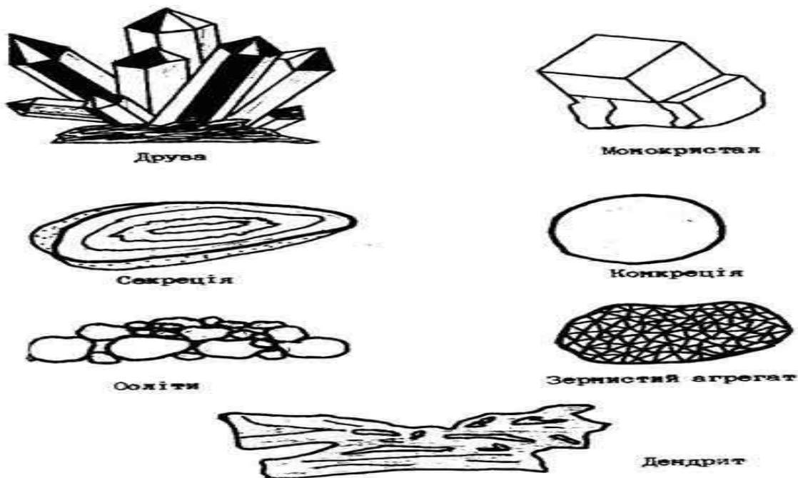
Рисунок 2.3—Форми знаходження мінералів у природі
