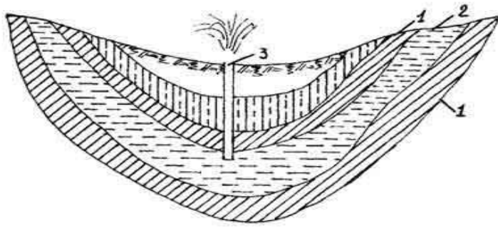
Рисунок 6.5 — Артезіанські води:
