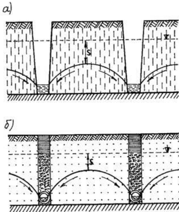
Рисунок 6.15 — Дренажні траншеї: а – відкриті; б – закриті
