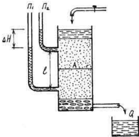
Рисунок 6.10 — Схема приладу для визначення коефіцієнта фільтрації пісків
