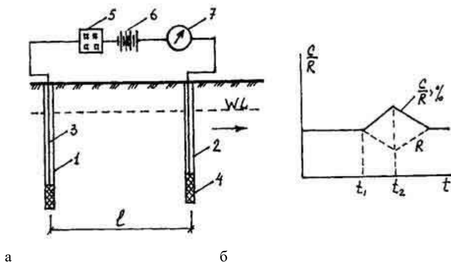
Рисунок 6.12 — Схема для визначення швидкості фільтрації:
