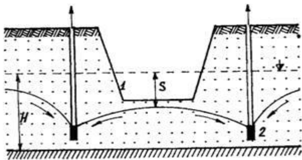
Рисунок 6.16 — Осушення будівельного котловану голкофільтрами: 1 – будівельний котлован; 2 – голкофільтри
