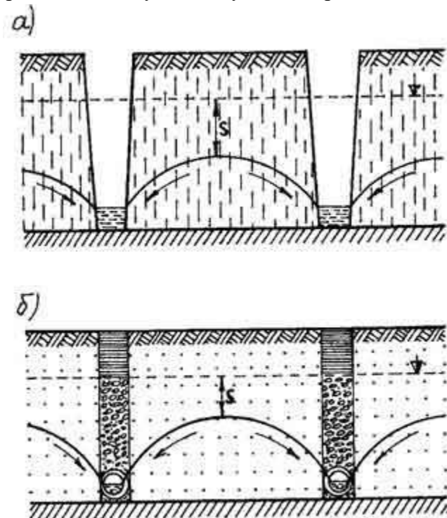
Рисунок 6.14 — Приплив води до досконалої свердловини:
