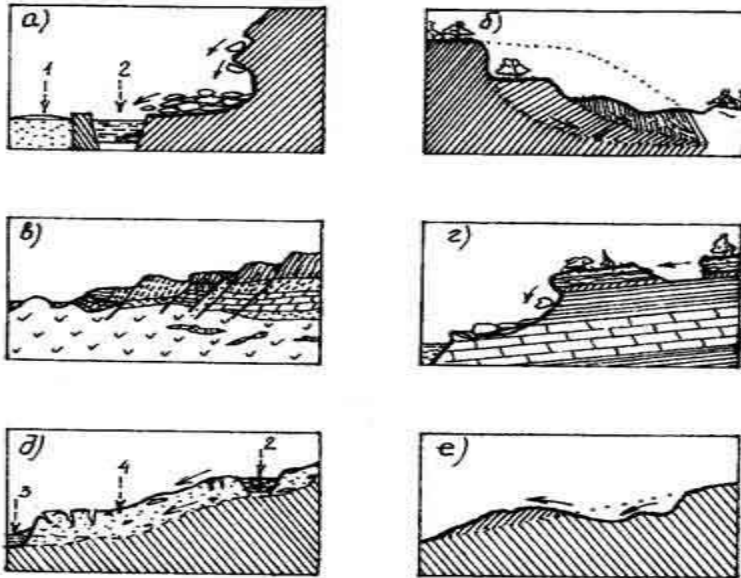
Рисунок 8.3 — Основні форми порушення стійкості і деформації схилів: а — обвали, вивали; б — обрушення із зрізом та обертанням; в — скол при просіданні; г — сковзання; д — покривні зсуви (сповзання); е — обпливання; 1 — шлях; 2 — канал; 3 — річка; 4 — зсувний делювій
