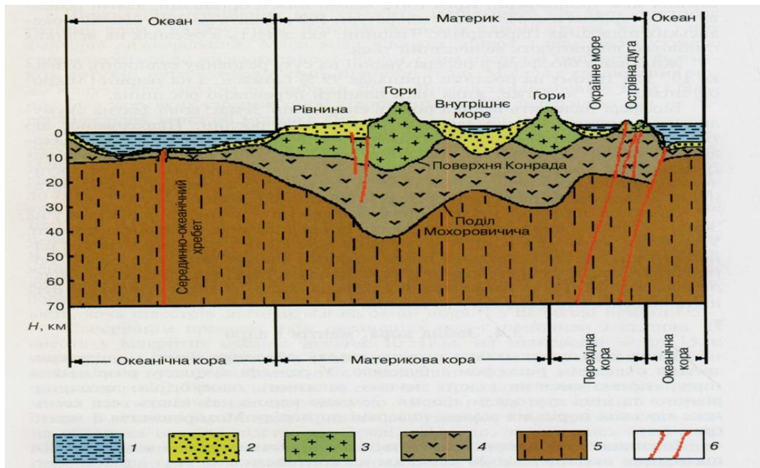
Рисунок 1.2 – Будова земної кори:
