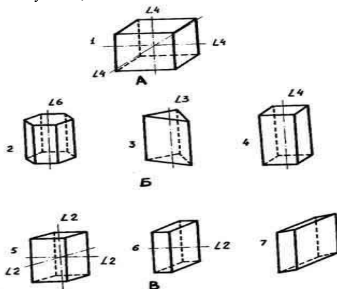
Рисунок 2.2 —Кристалографічні сингонії:
