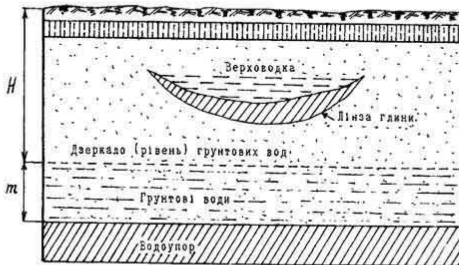
Рисунок 6.3 — Ґрунтові води
