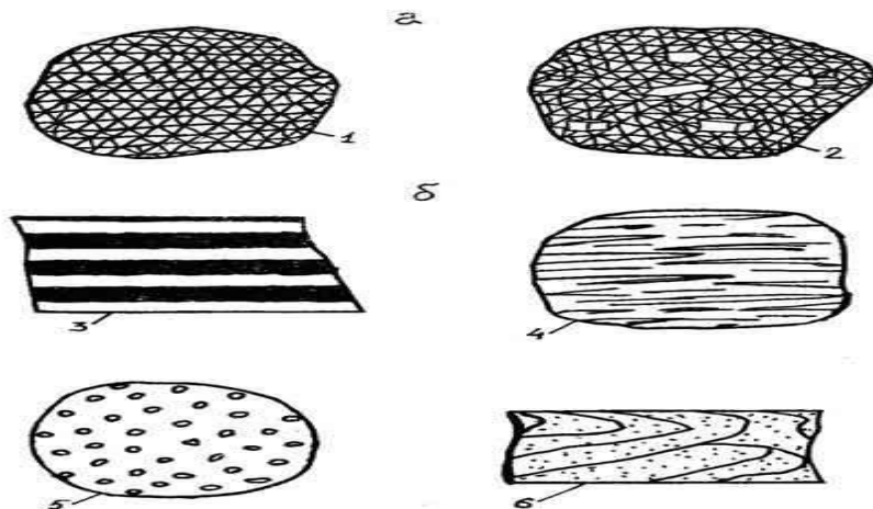
Рисунок 4.1—Структура та текстура гірських порід:
