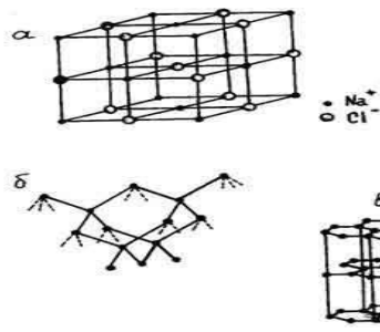
Рисунок 2.1 —Будова кристалічних решіток: а – галіту; б – алмазу; в – графіту
