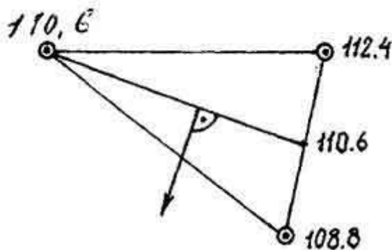
Рисунок 6.11 — Схема визначення напрямку руху ґрунтових вод
