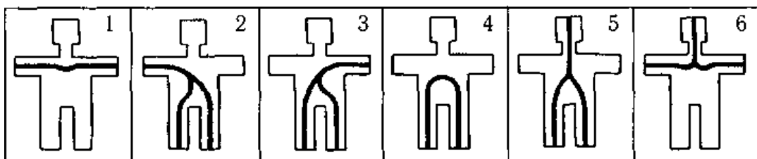
Рис. 7.3. Найбільш поширені шляхи проходження струму через тіло людини: 1 — рука—рука»; 2 — «права рука—ноги»; 3 — «ліва рука—ноги»; 4 — «нога—нога»; 5 — «голова—ноги»; 6 — «голова—руки»
