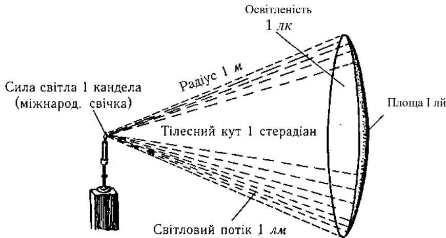
Рис. 4.1. Схема, що пояснює деякі основні світлотехнічні одиниці
