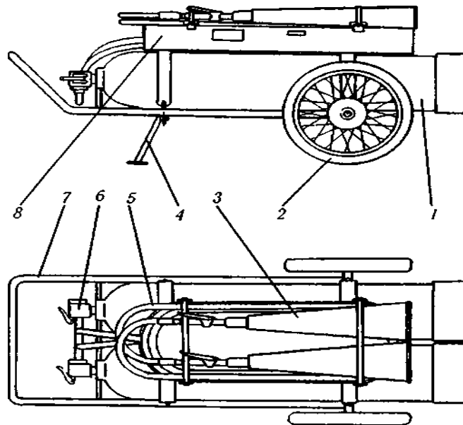
Рис. 9.2. Пересувний вогнегасник ВВ-80:
