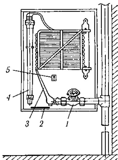
Рис. 9.4 Внутрішній пожежний кран
