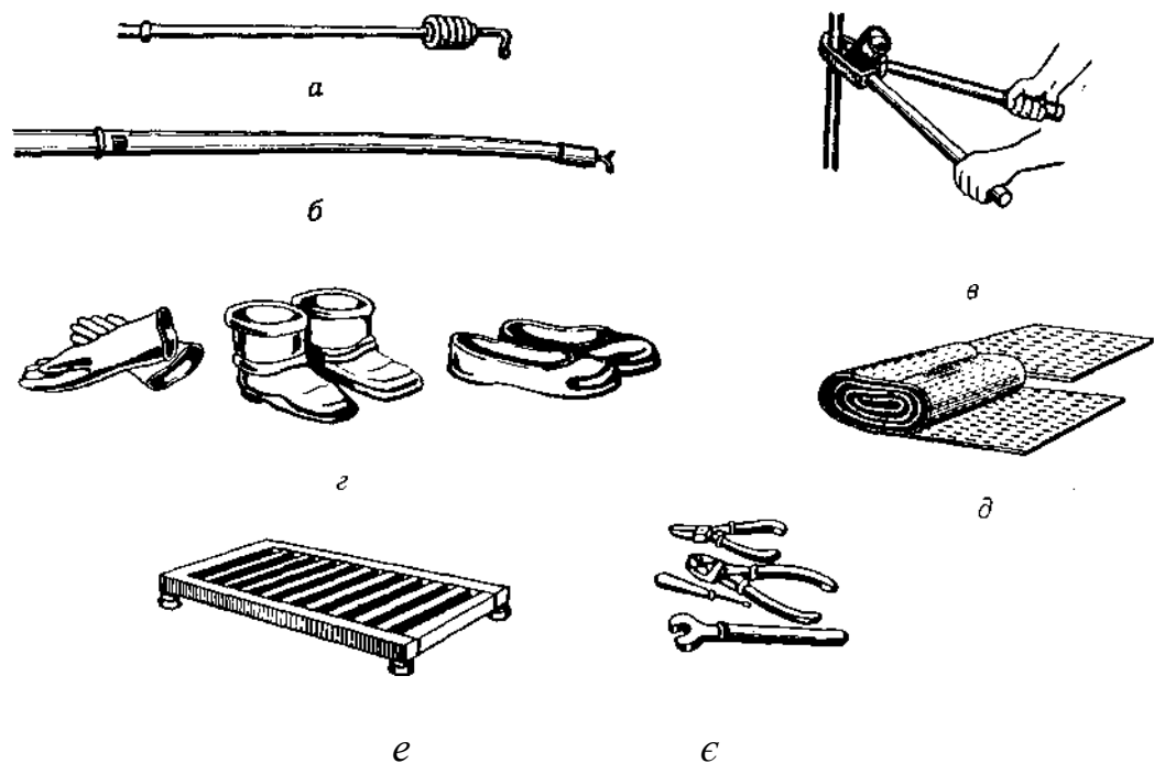
Рис. 7.4. Ізолювальні електрозахисні засоби: а — ізолювальна штанга; б — показчик напруги; в — струмовимірювальні кліщі; г — діелектричні рукавички, боти, калоші; д — гумові килимки та доріжки; е — ізолювальна підставка; є — інструменти з ізолюваними ручками
