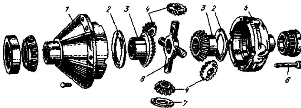
Мал.24.4 Конічний симетричний диференціал
