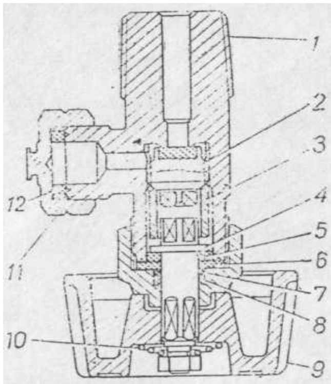
Рис. 3. Наповнюючий вентиль:
