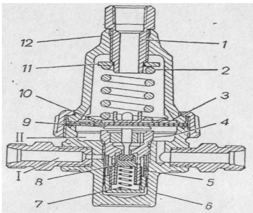
Рис. 4. Редуктор високого тиску:
