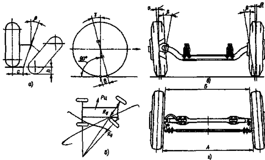
Мал.26.2 Кути встановлення передніх коліс автомобіля
