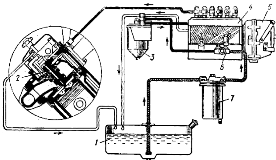
Рис. 1. Принципова схема системи живлення дизельного двигуна:
