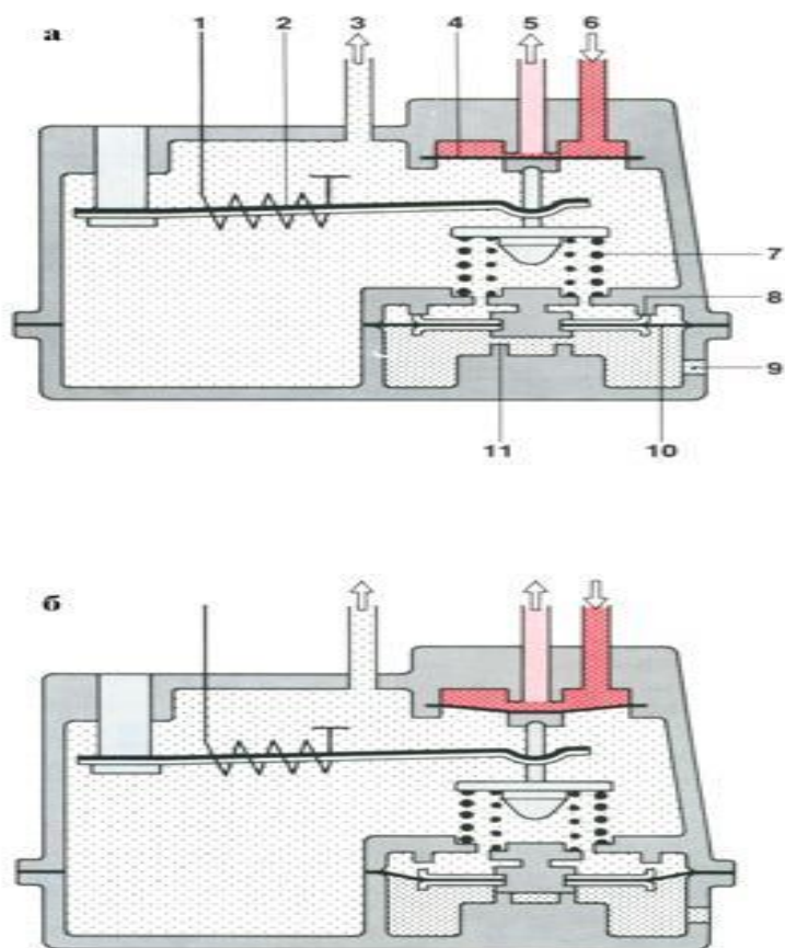
Рис. 22. Регулятор керуючого тиску:
