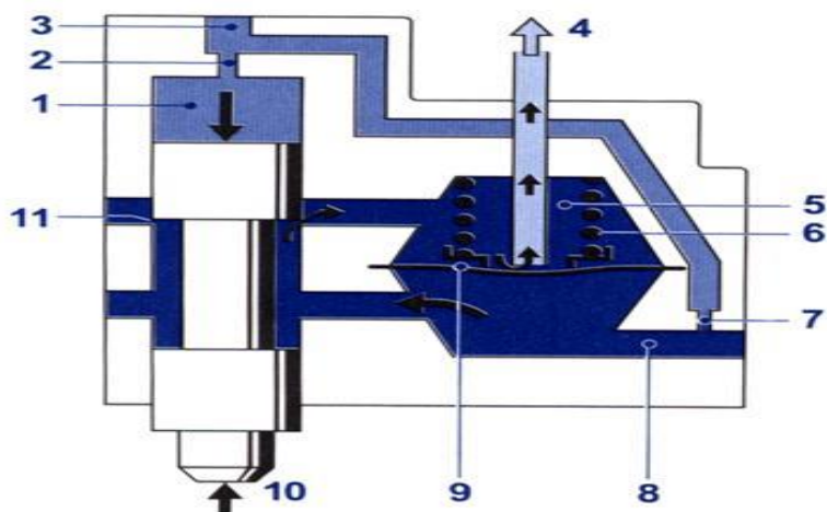
Рис. 18. Конструкція диференціального клапана, пов'язаного з контурами керуючого тиску і тиску в системі:
