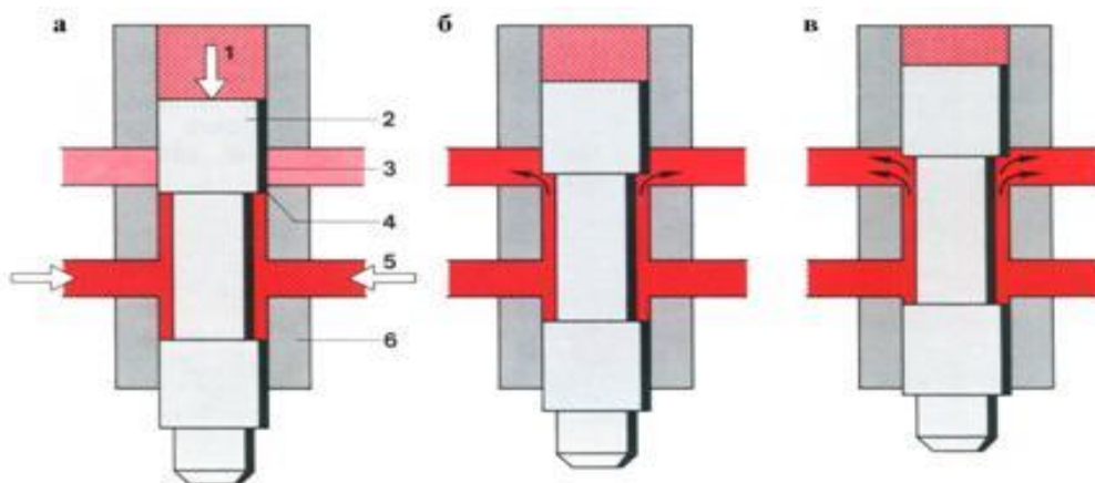
Рис. 16. Розподільник і гільза з дозуючими щілинами:
