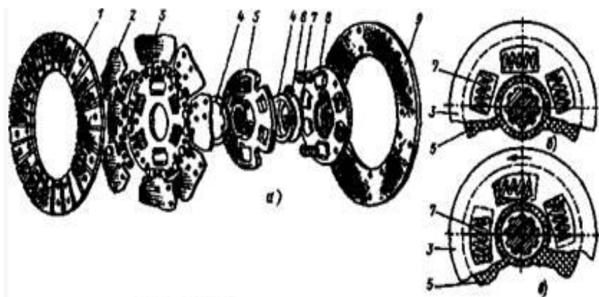
Мал.19.2 Гаситель крутильных колебаний
