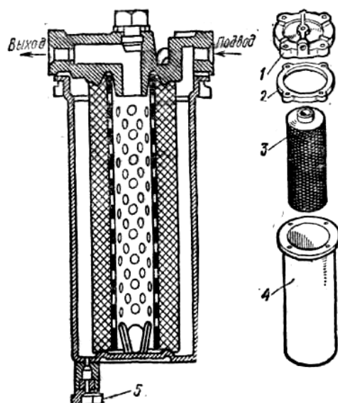
Рис. 2. Фільтр грубого очищення палива:
