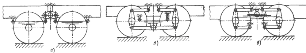
Рис. 6. Схеми балансирних підвісок
