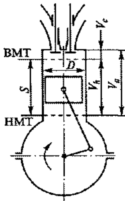
Рис. 2. Основні параметри двигуна
