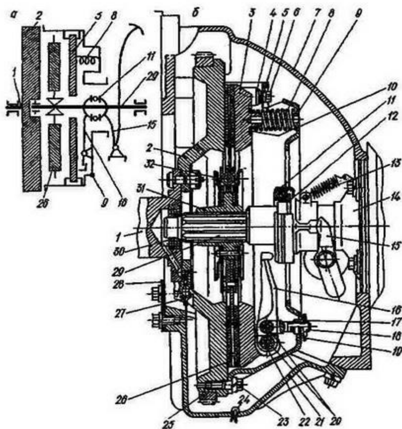
Мал.19.1 Схема і конструкція однодискового зчеплення автомобіля ЗІЛ-130
