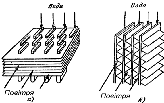
Мал. 3. Охолоджуючі серцевини радіаторів: а - трубчасто-пластинчастого; б - трубчасто-стрічкового
