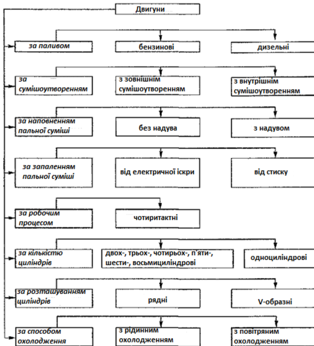
Рис. 1. Основні типи автомобільних двигунів, класифікованих за різними ознаками
