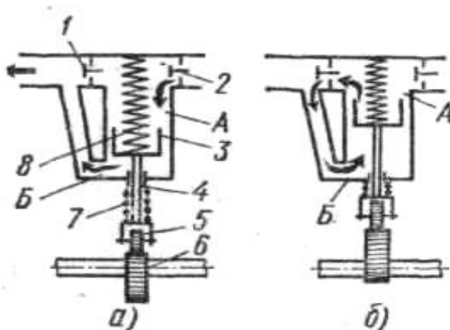
Рис. 5. Схема роботи паливоподаючого насоса:
