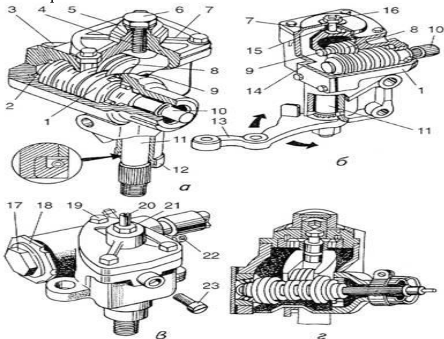
а — «Москвич»; б — ВАЗ; в — ЗАЗ; г — ГАЗ-24; 1 — черв'як; 2 — регулювальна гайка; 3, 4, 21 — контргайки; 5 — регулювальна муфта; 6, 19 — пробки оливозаливних отворів; 7 — кришка картера; 8 — ролик; 9 — вісь ролика; 10 — рульовий вал; 11 — вал рульової сошки; 12 — сальник; 13 — рульова сошка; 14 — регулювальні прокладки; 15 — прокладка регулювального гвинта; 16, 20 — регулювальні гвинти; 17 — регулювальна пробка; 18 — стопорна гайка; 22 — болт стяжного хомута; 23 — болт контрольного отвору рівня оливи
