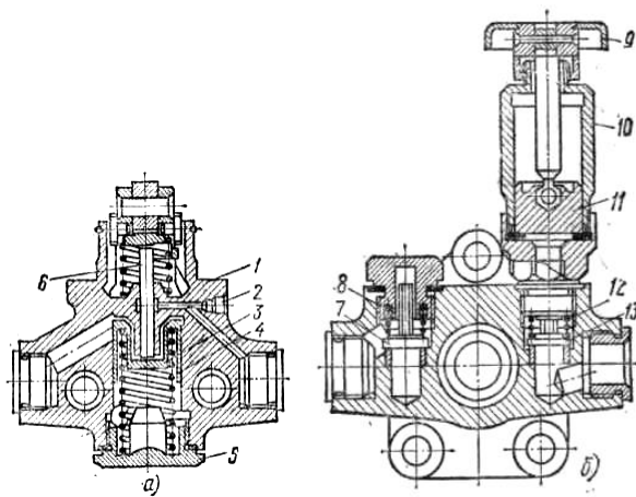
Рис. 4. Паливоподаючий насос:
