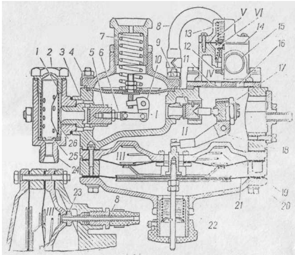
Рис. 7 Газовий редуктор низького тиску:
