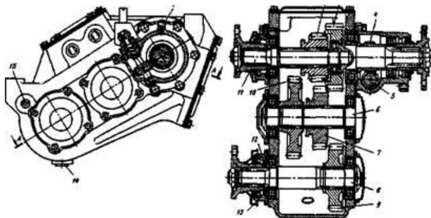
Мал.22.1 Роздавальна коробка
