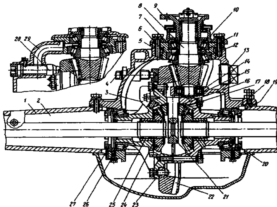
Мал.24.2 Одинарна головна передача
