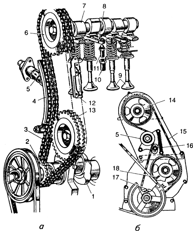
Рис. 2. Приводи розподільного вала:
