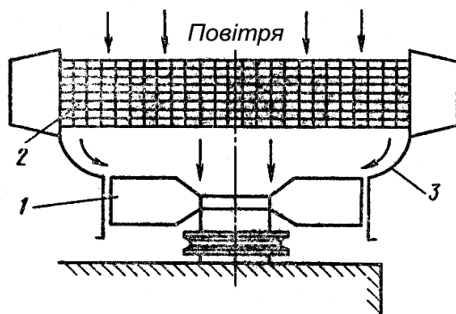
Мал. 4. Схема повітряного тракту з направляючим кожухом: 1-вентилятор; 2 - радіатор; 3 - кожух.
