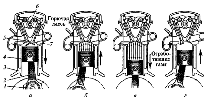
Рис. 2.3. Схема робочого процесу чотиритактного бензинового двигуна:
