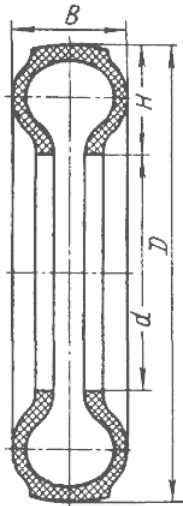
Рис. 2. Основні розміри автомобільної шини
