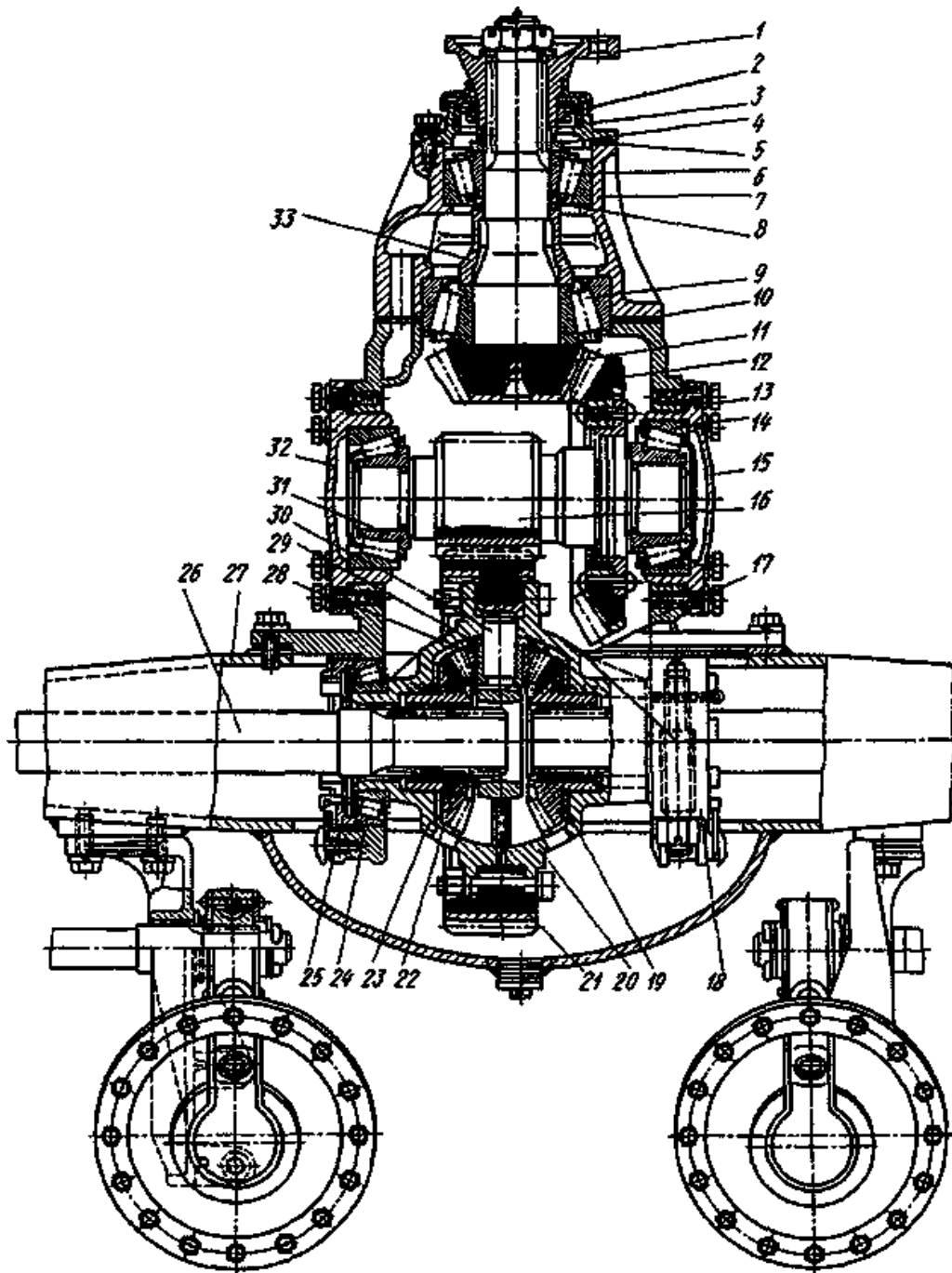
Мал.24.3 Подвійна головна передача
