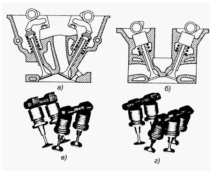
Рис. 4. Привод клапанів двома розподільними валами:
