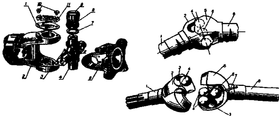
Мал.23.2 Карданний шарнір нерівних кутових швидкостей
