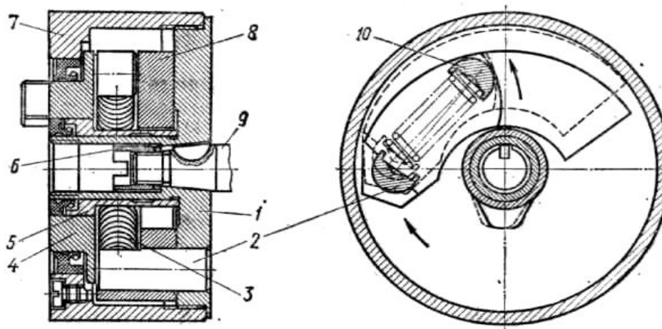
Рис. 9. Муфта автоматичного випередження упорскування палива
