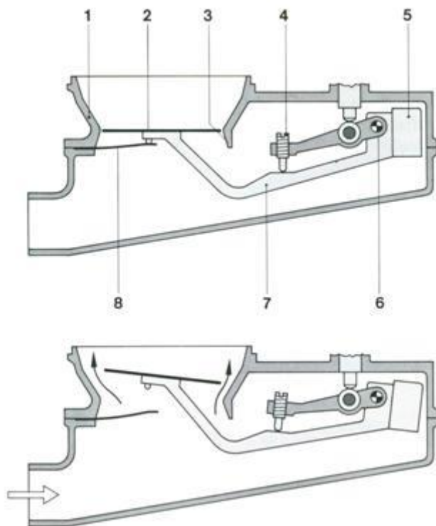
Рис. 14. Витратомір повітря:
