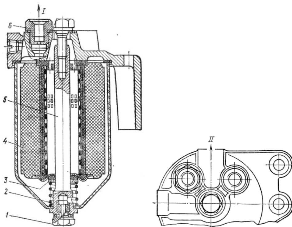
Рис. 3. Фільтр тонкого очищення палива:
