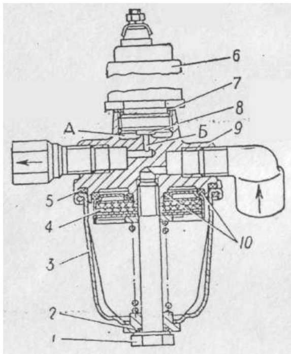
Рис. 5. Електромагнітний клапан з фільтром для газу:
