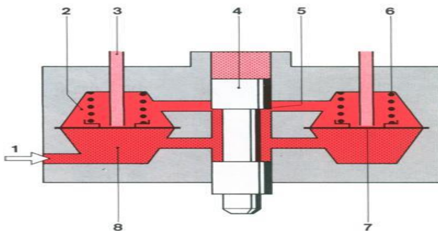
Рис . 19. Дозатор палива з диференціальними клапанами:
