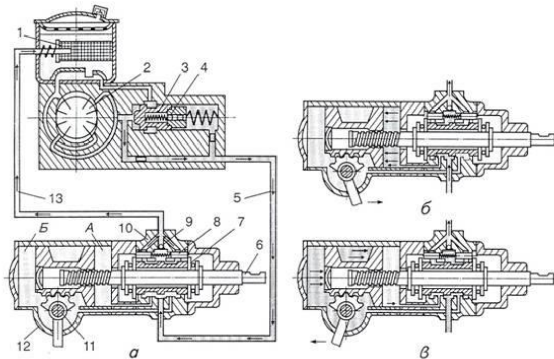
Рис. 6. Схема роботи гідро підсилювача:
