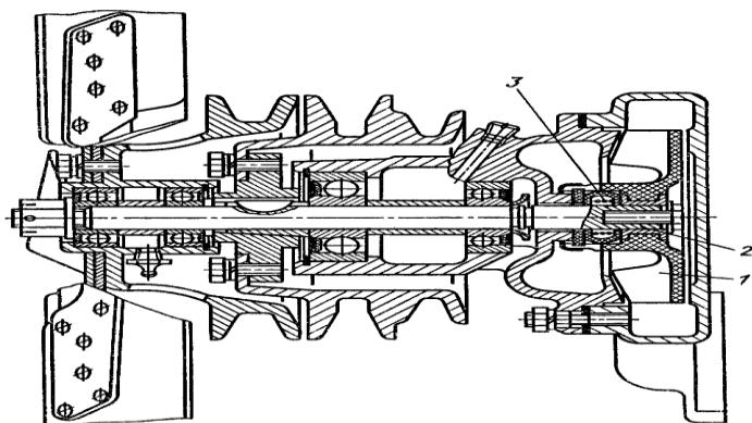
Мал. 2. Водяний насос двигуна ЗІЛ-131:
