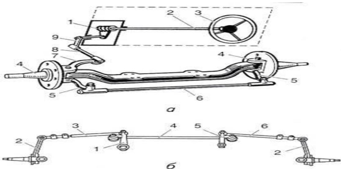
Рис. 2. Схеми рульового керування:
