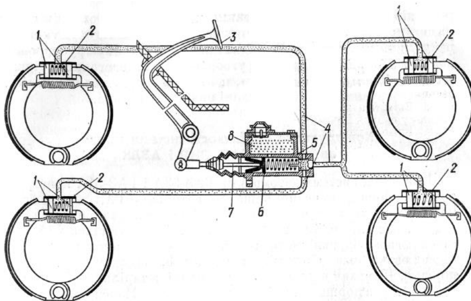
Рис. 136. Схема гальмівної системи з гідравлічним приводом гальм: 1 — поршні колісних гальмівних циліндрів; 2 — колісні гальмівні циліндри; 3 — гальмівна педаль; 4 — трубопроводи; 5 — головний гальмівний циліндр; 6 — поршень; 7 — шток; 8 — резервуар.
