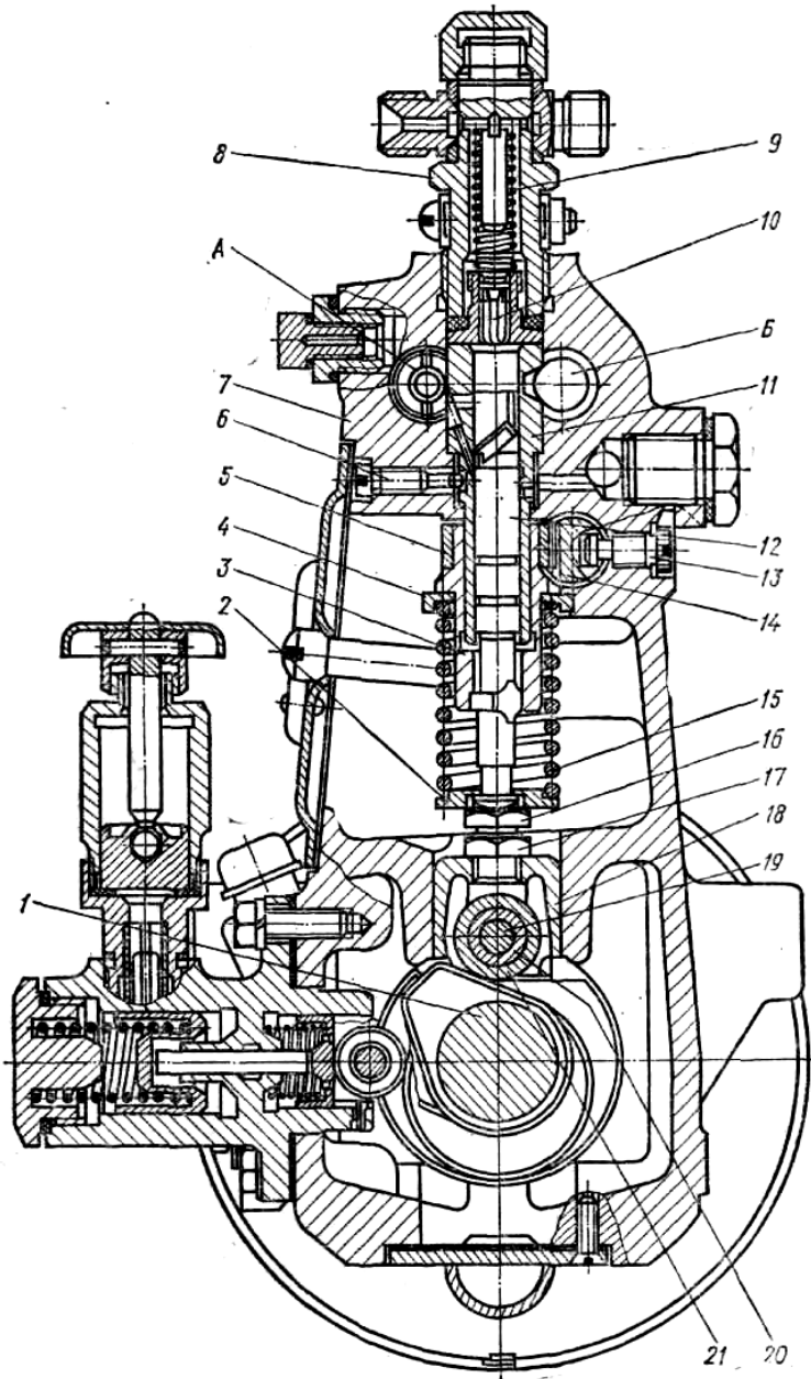
Рис. 6. Поперечний розріз насоса високого тиску:
