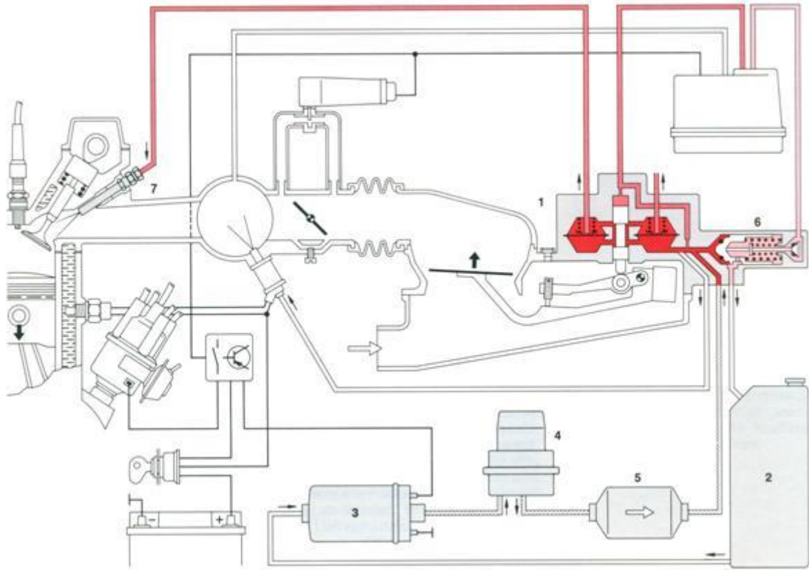
Рисунок 3. Схема роботи системи К-Джетронік при пуску двигуна:
