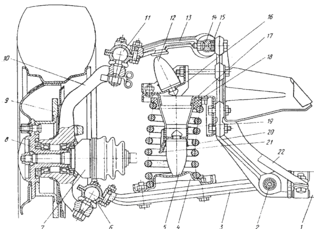
Рис. 8. Незалежна пружинна важільна підвіска керованих і ведучих коліс (ВАЗ-2121)
