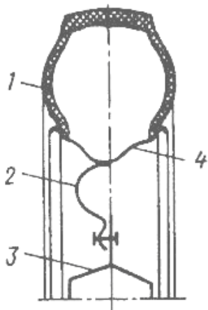
Рис. 1. Схема автомобільного колеса
