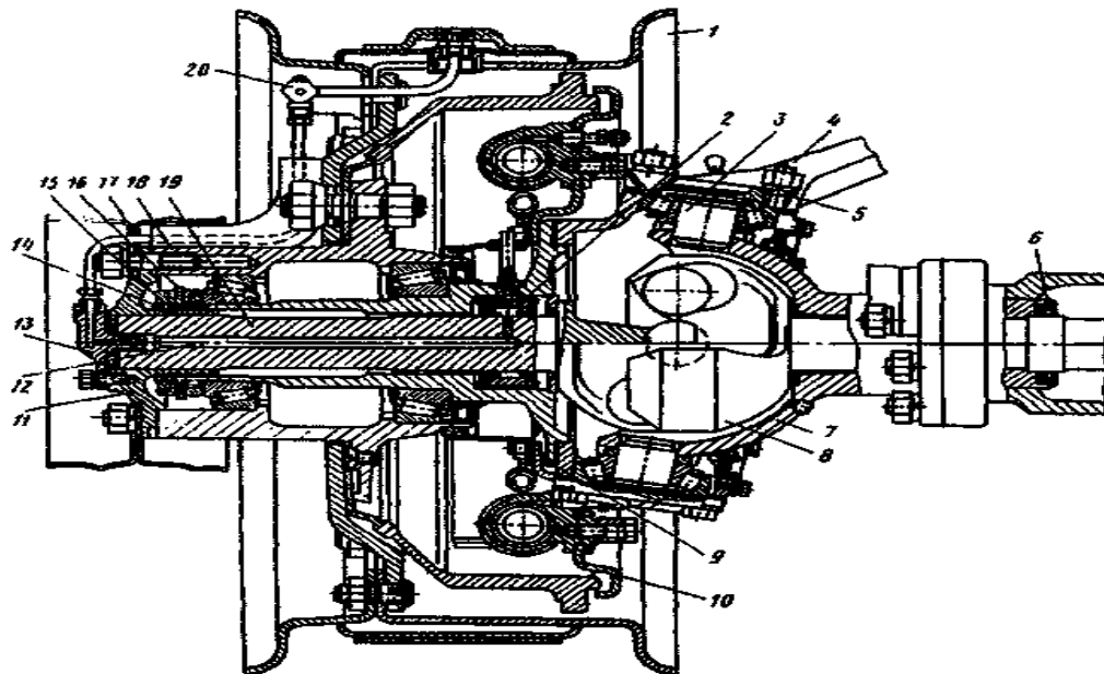
Мал.23.3 Карданний шарнір рівних кутових швидкостей
