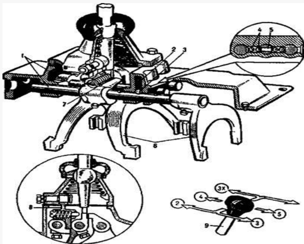
Мал.21.2 Механізм переключення передач коробки зміни передач
