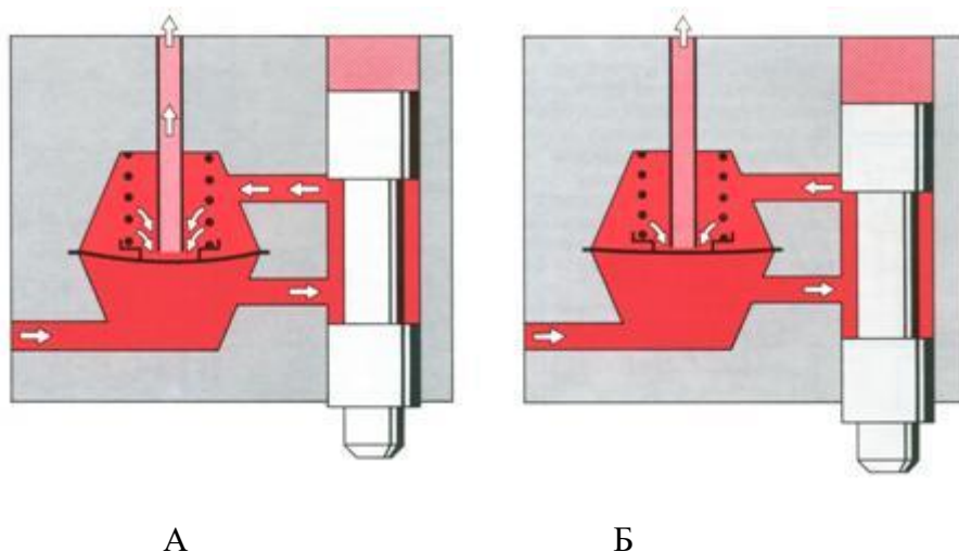
Рис. 20. Схема роботи диференціальних клапанів:
