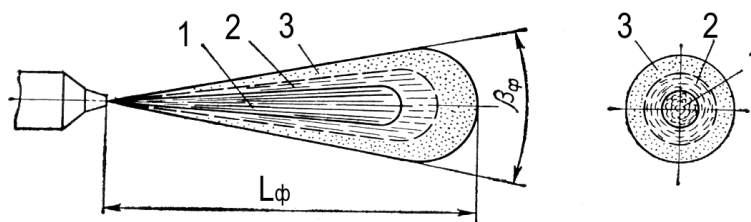
Рис. 1. Структура факела розпилення палива
