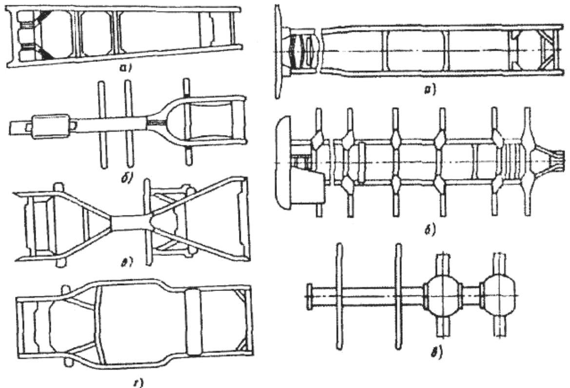
Рис. 3. Схеми рам легкових автомобілів (зліва): а — драбинна; б — хребтова; в — Х-подібна; г — периферійна
