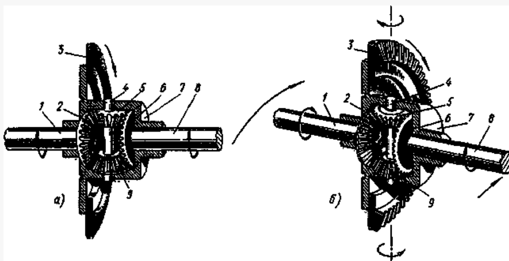
Мал.24.5 Схема роботи диференціала
