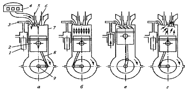
Рис. 4. Схема робочого процесу чотиритактного дизеля: а - впускання, б - стиснення; в - робочий хід; г - випуск; 1 - паливний насос; 2 - поршень, 3 - форсунка; 4 - повітряний фільтр; 5 - впускний клапан; 6 - випускний клапан; 7 - циліндр; 8 - шатун; 9 - колінчастий вал
