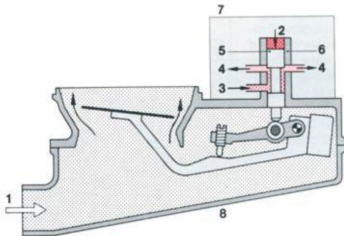
Рис . 15. Схема роботи дозатора палива:
