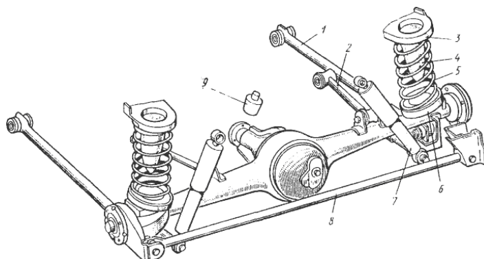
Рис.7. Задня залежна підвіска легкового автомобіля на спіральних пружинах (ВАЗ-2105)
