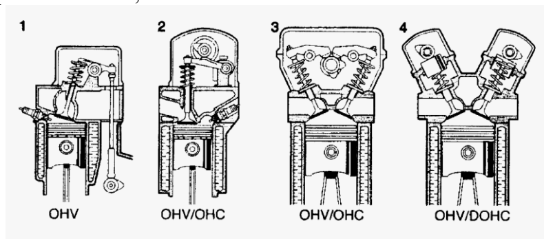
Рис. 1. Конструктивні варіанти привода клапанів
