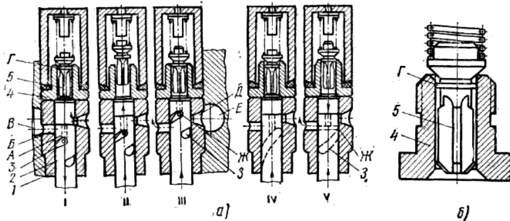
Рис. 7. Плунжер форсунки:
