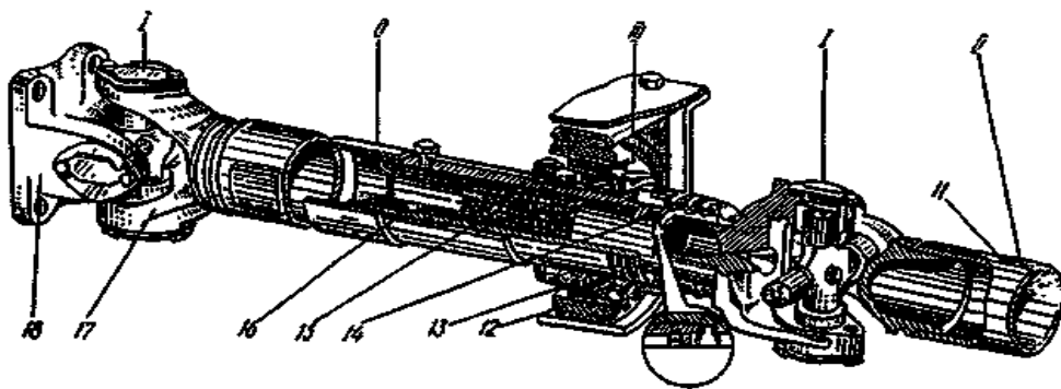
Мал.23.1 Карданна передача
