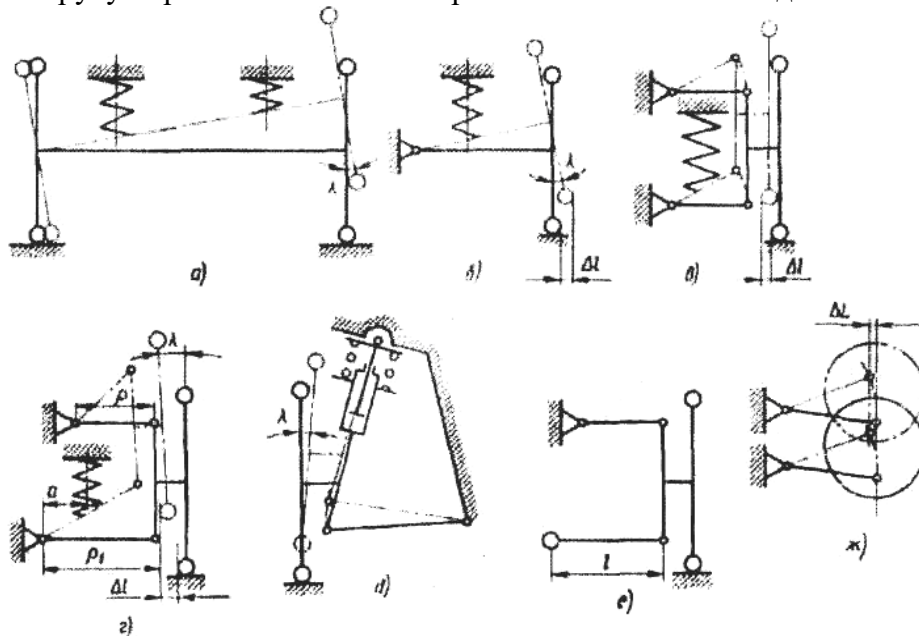
Рис. 5. Кінематичні схеми основних типів підвісок: а — залежна; б — незалежна однаважільна; в, г — незалежна з важелями, відповідно, рівної та нерівної довжини; д — незалежна важільно-телескопічна (типу Мак-Ферсон); е — незалежна двоважільна з торсіоном; ж — незалежна з подовжньою площиною коливань
