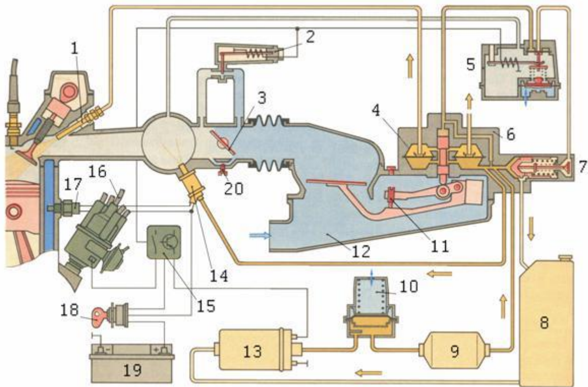
Рис. 2. Конструктивна схема системи упрскування палива К-Джетронік:
