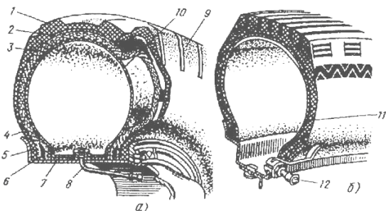
Рис. 1. Конструкція автомобільної шини: а — камерної; б — безкамерної
