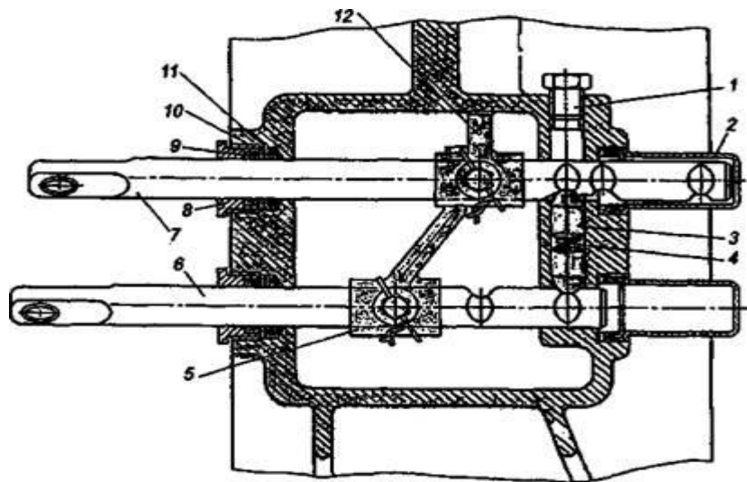
Мал.22.2 Механізм переключення передач роздавальної коробки
