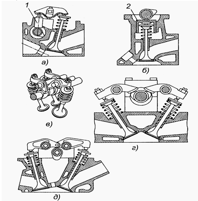
Рис. 3 Привод клапанів одним розподільним валом: а, б - при однорядному розміщенні клапанів; в - д - при дворядному розміщенні клапанів; 1 - гідрокомпенсатор; 2 - направляючий стакан
