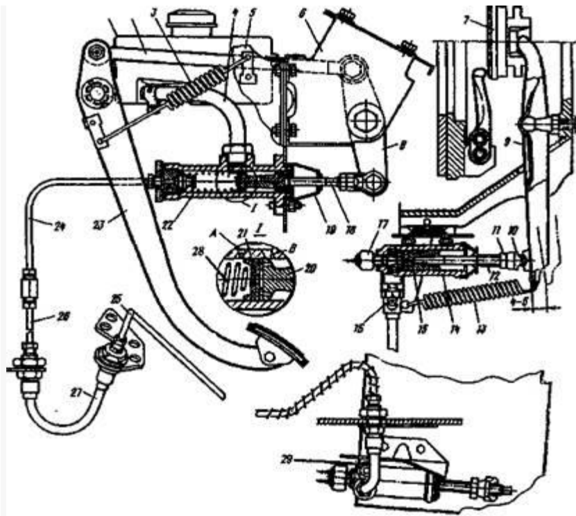
Мал.20.2 Привод виключення зчеплення автомобілів ГАЗ-66-11
