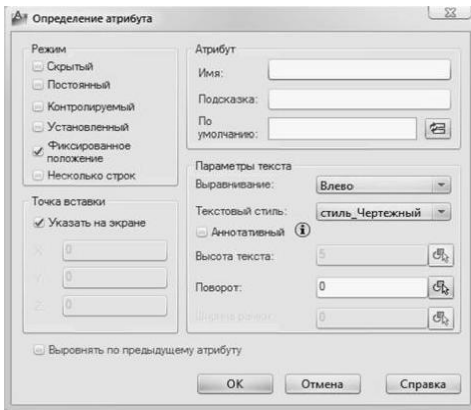
Рис. 5.7. Діалогове вікно команди „Attdef (Атопр)”
