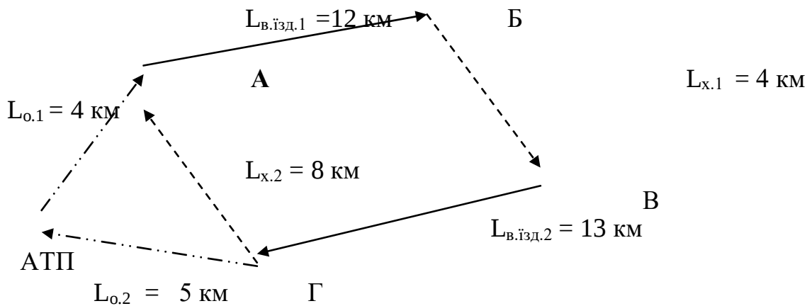
Мал. 9 Схема кільцевого маршруту.
