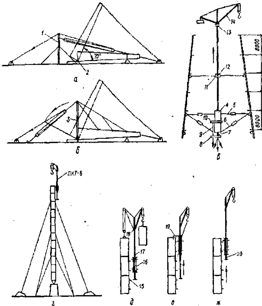
Мал. 12. Спорудження веж та щогл: а – монтаж веж висотою до 100 м у зібраному вигляді
