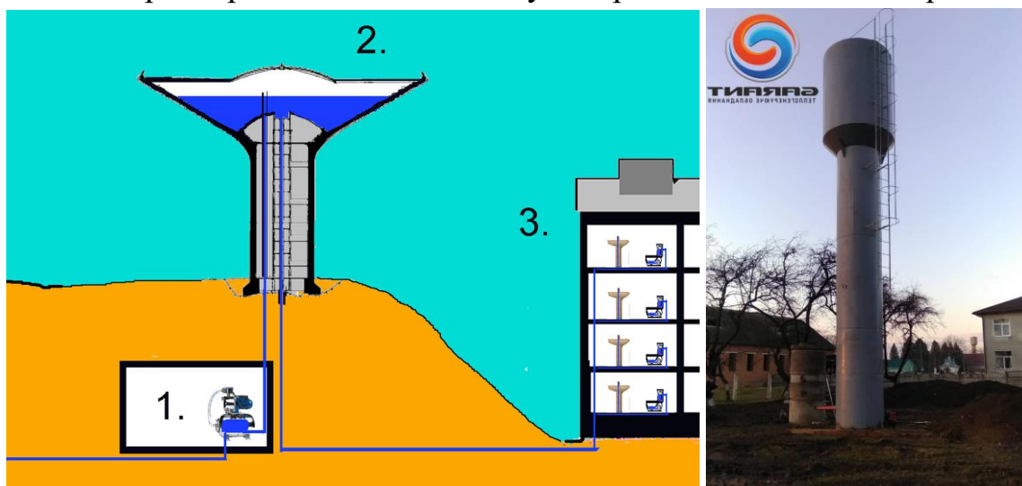
Мал.9. Водонапірна вежа
