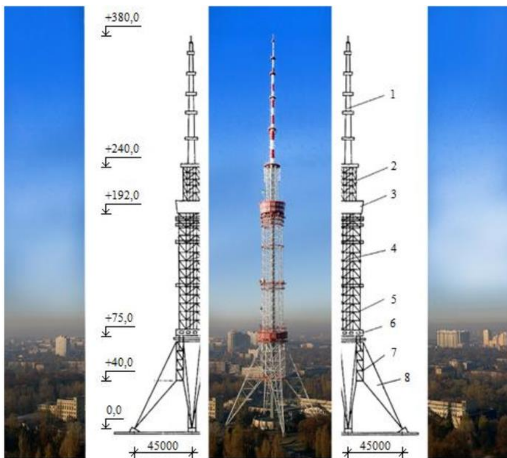
Мал. 14. Київська телевізійна вежа
