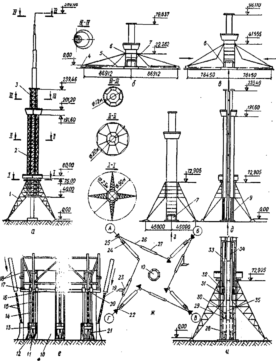
Мал. 13. Спорудження телевізійної вежі підручанням:
