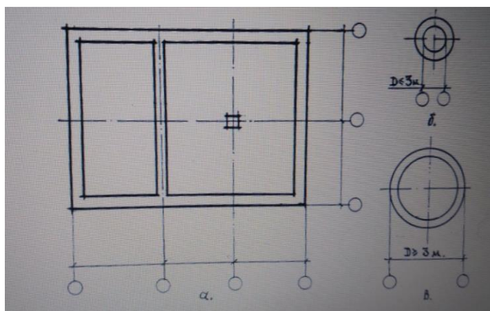
Мал.2. – Прив'язка розбивочних вісей до конструкцій споруд а – прямокутних; б, в – циліндричних відповідно d \leq 3 м і d > 3 м.
