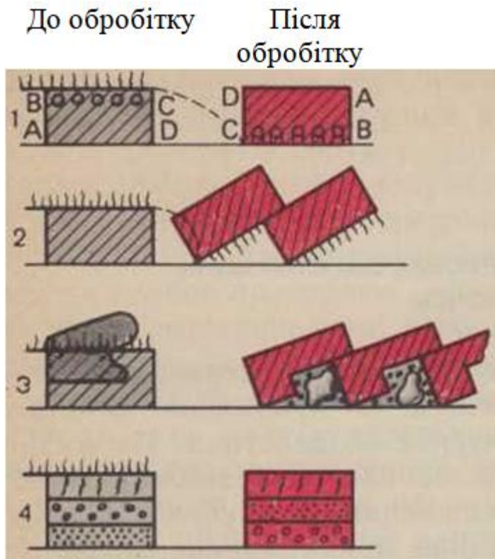
Рис. 3.3.1. Основні операції оранки:
