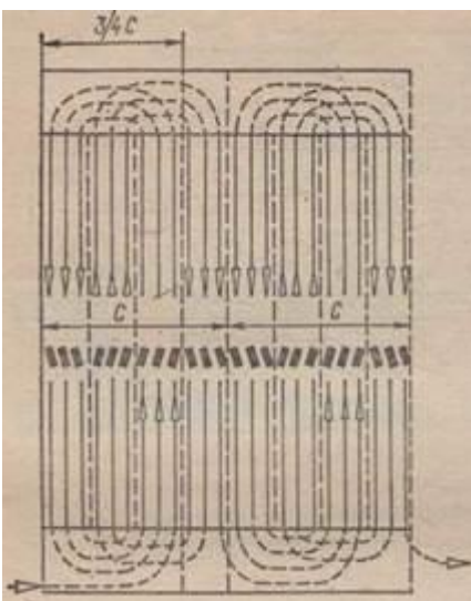
Рис. 3.3.9. Безпетльовий комбінований спосіб руху
