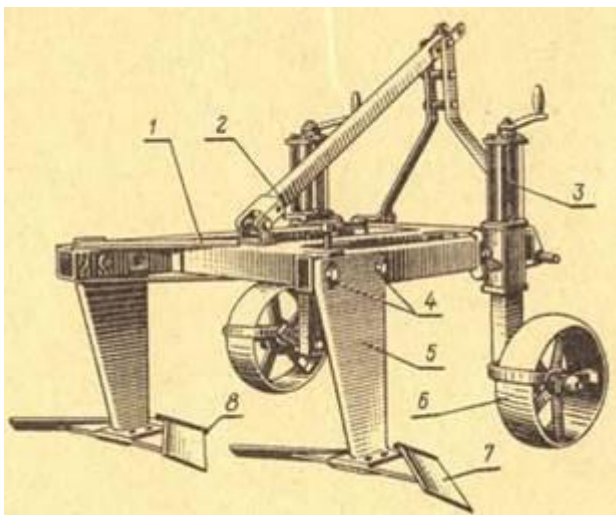
Рис. 3.3.2. Культиватор-плоскоріз КПГ-250
